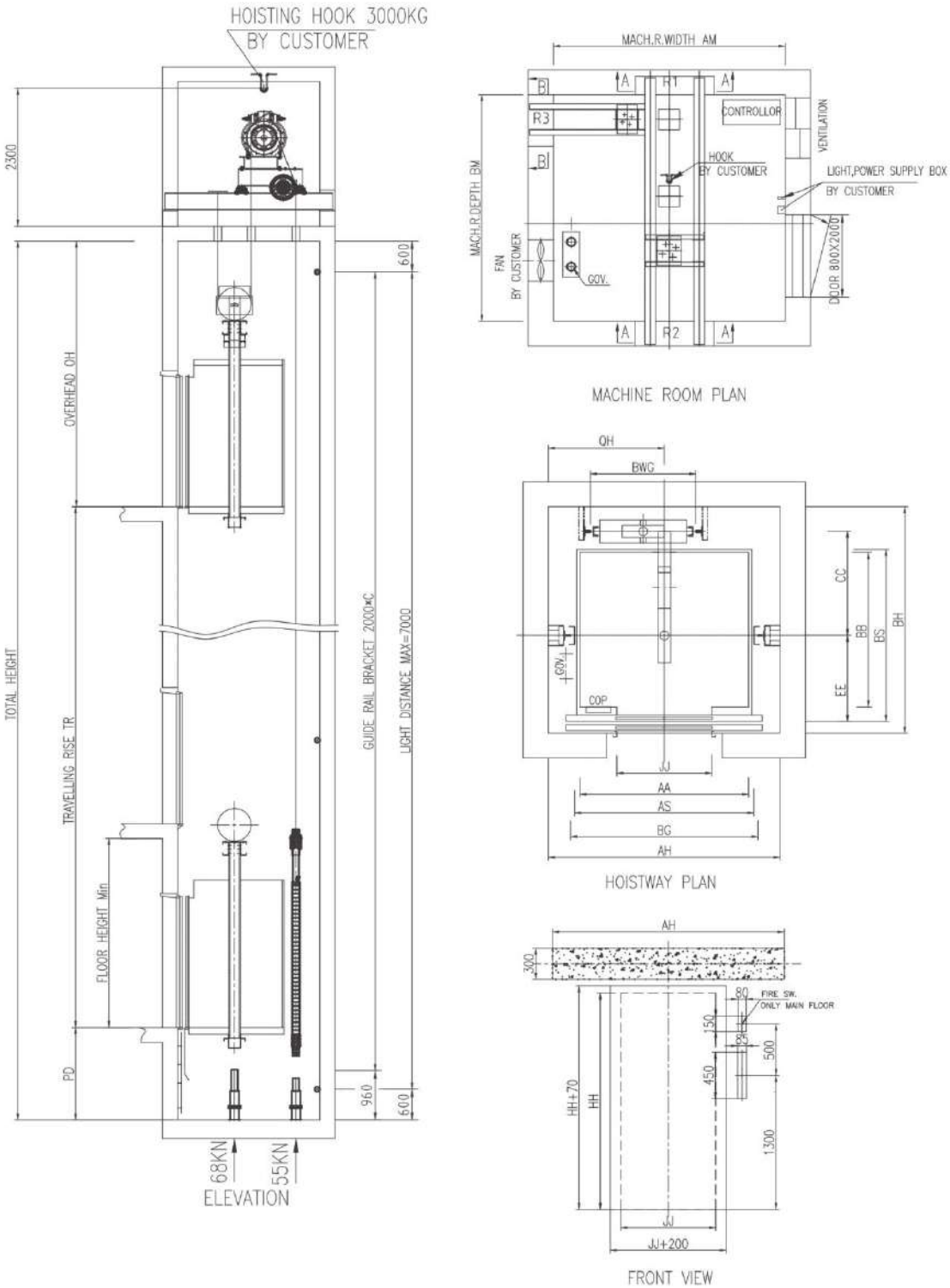
INACHI ELEVATOR Mini MR passenger elevator
